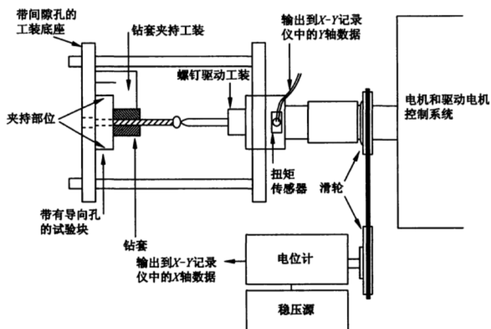
图 1 旋动扭矩试验装置
